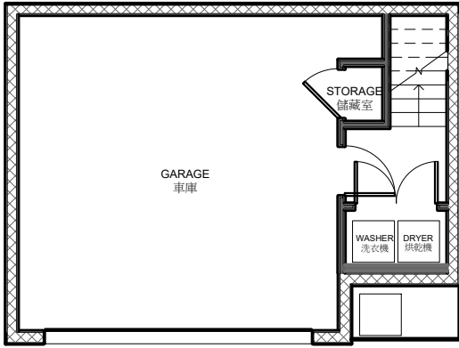
GARAGE 車庫 407 S.F.
