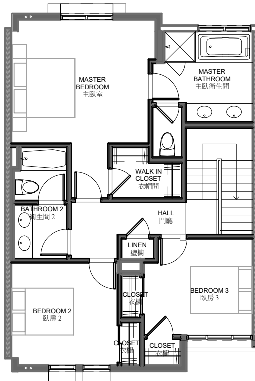
Second Floor Plan 975 S.F. 二樓平面圖
