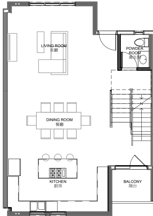
First Floor Plan 913 S.F. 一樓平面圖
