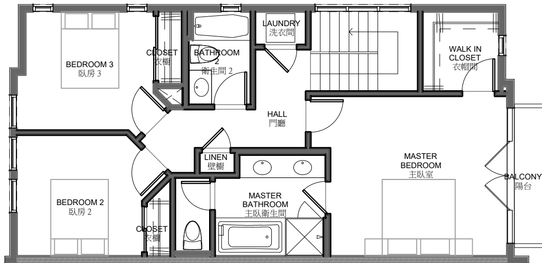
Second Floor Plan 966 S.F. 二樓平面圖
